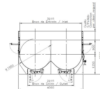
SECCIÓN A-A
